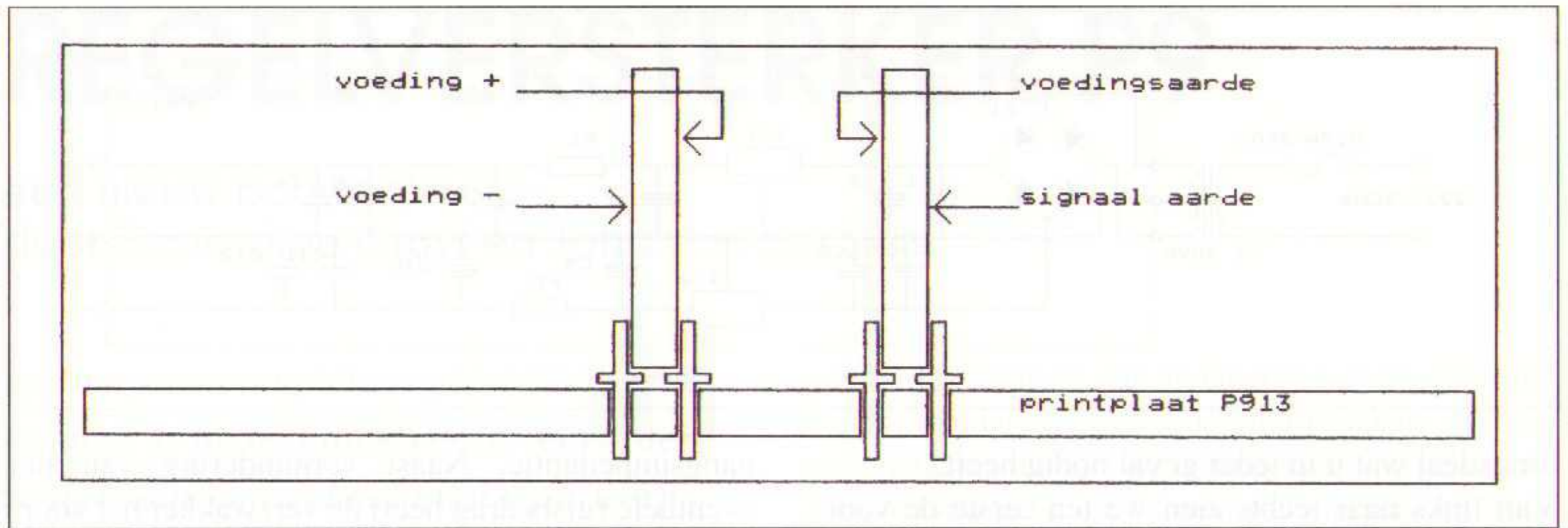
Figuur 4. Aarde- en voedingsbanen.
